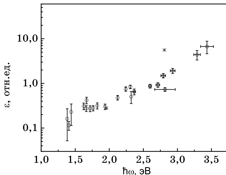
Рис. 5. Зависимость эффективности возбуждения полосы ФИП на 1.6 эВ в расчете на поглощенный фотон возбуждения от его энергии (спектр фотовозбуждения), температура \approx 85 К. Две точки (*) соответствуют данным рис. 4.
