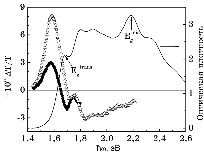
Рис. 4. Спектры ФИП при лазерном возбуждении с энергией фотона 2.81 эВ ( \Delta ) и 1.96 эВ ( \bullet ), интенсивностях возбуждения \simeq 0.2 и 0.6 Вт/см 2 , соответственно, частоте модуляции 140 Гц и комнатной температуре. Сплошной линией показан спектр линейного поглощения, на котором отмечены бесфононные пики поглощения транс и цис-изомеров НПА.
