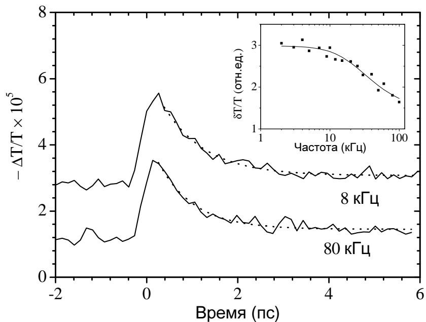
Рис. 6. Модуль сигнала ФИП на 1.55 эВ как функция времени задержки между импульсами зондирования и возбуждения для двух частот модуляции. Экспоненциальные кинетики с временными константами 0.9 и 0.8 пс показаны пунктирными линиями для частот модуляции 8 и 80 кГц, соответственно. На вставке показан модуль сигнала ФИП на 1.55 эВ как функция частоты модуляции, сплошная линия соответствует мономолекулярной кинетике с характерным временем 7 мкс.
