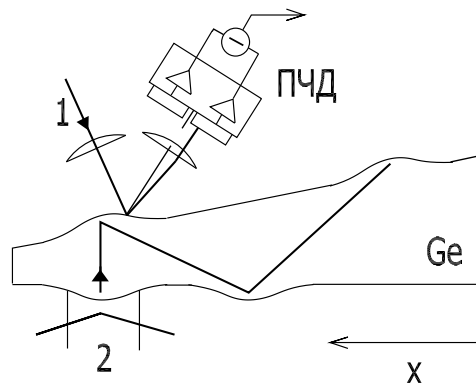
Рис. 2. Геометрия эксперимента с клиновидными образцами (угол клина 1.5-3^\circ ). Пучок возбуждения (2) генерирует акустический импульс, распространяющийся в образце, профиль и временное положение которого измеряются с помощью пучка зондирования (1), используя фотодефлекционную методику и позиционно-чувствительный детектор (ПЧД). Перемещение клина вдоль оси X позволяет измерять профили акустических импульсов при различных длинах распространения.
