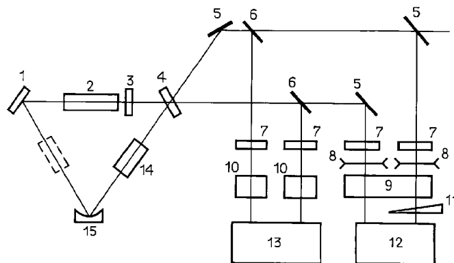
Рис. 1. Принципиальная схема экспериментальной установки: 1, 4 — плоские зеркала кольцевого резонатора, 2 — кристалл рубина, 3 — просветляющий фильтр, 5 — поворотные зеркала, 6 — светоделительные элементы, 7 — светофильтры, 8 — линзы, 9 — интерферометр Фабри-Перо, 10 — фотоприемники, 11 — оптический клин, 12 — фотоаппарат, 13 — двухлучевой осциллограф, 14 — камера со сжатым водородом, 15 — сферическое зеркало кольцевого резонатора
