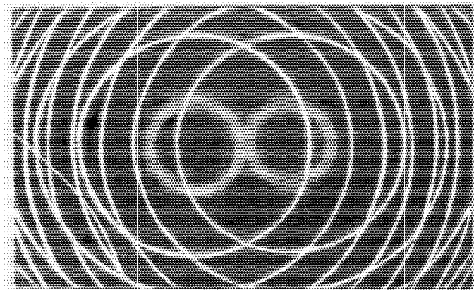
Рис. 3. Спектрограммы встречных волн (база интерферометра Фабри-Перо 0,5 см)
