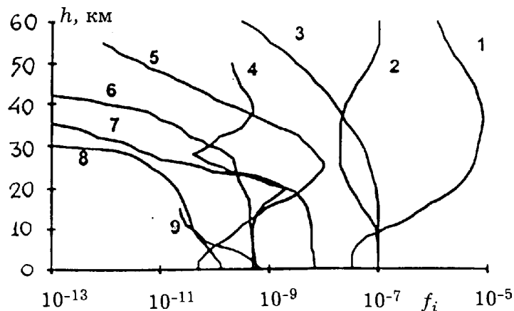
Рис. 1. Высотные распределения фоновых относительного содержания ряда МГС: 1 — O_3 , 2 — CO , 3 — N_2O , 4 — ClO , 5 — HNO_3 , 6 — COS , 7 — NH_3 , 8 — SO_2 , 9 — H_2CO
