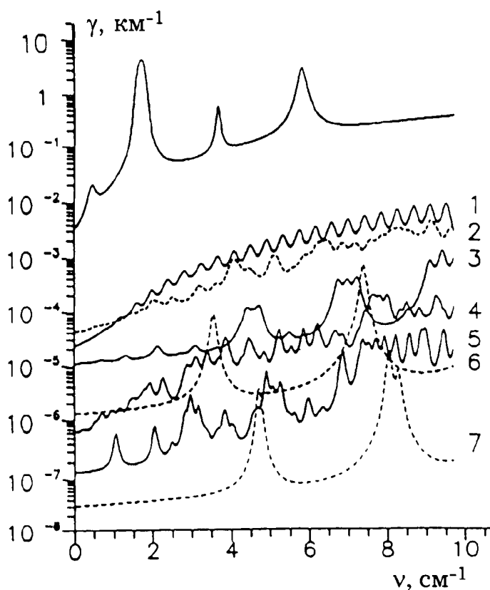
Рис. 2. Коэффициенты поглощения примесных компонент (1 — HNO_3 , 2 — SO_2 , 3 — H_2CO , 4 — O_3 , 5 — NO_2 , 6 — CO , 7 — NO ) при стандартных атмосферных условиях на уровне моря (давление P = 760 мм рт. ст., температура T = 293 К) и содержании, соответствующем ПДК. Верхняя кривая — суммарный коэффициент поглощения водяного пара и молекулярного кислорода
