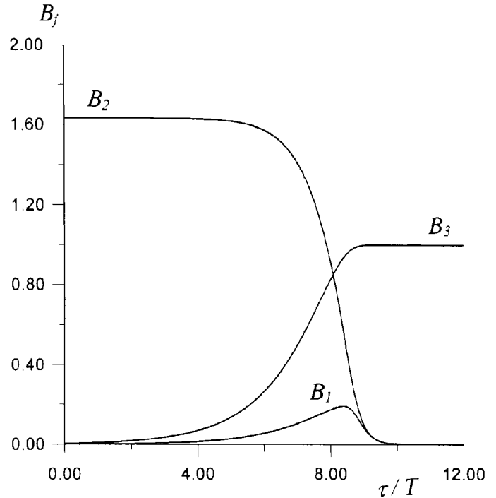
Рис. 1. Огибающие кинка и светлых солитонов при высокочастотной накачке в среде с \beta_2 = 4,9\beta_3 , u_1 = 1,5u_2 , u_3 = 0,5u_2 , u_2/u_c = 5 , E_3 = 1
