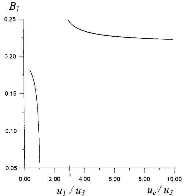
Рис. 2. Зависимости пиковой амплитуды солитона первой гармоники от скорости его распространения при E_3 = 1 , E_1 = 0,0001 и \beta_2/\beta_3 = 4
