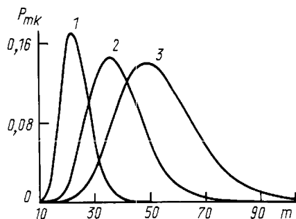
Рис. 1. Зависимость вероятности возникновения k = 10 эксимолей от количества диполей m при D_0/r_0 = 0,92 \cdot 10^{-19} Кл и I(\omega_{ex}) = 90 (1); 55 (2) и 40 кВт/см 2 (3)
