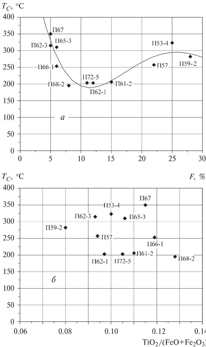
Рис. 2. Температуры Кюри T_c базальтов с различной степенью окисления F (а) и относительным содержанием TiO_2 (б)
