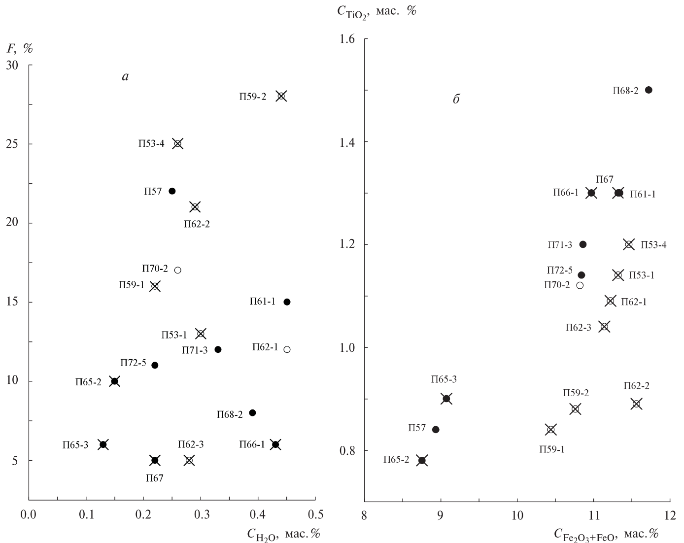
Рис. 1. Геохимические данные: а — соотношение между степенью окисления базальтов F и содержанием воды в них; б — соотношение между содержанием TiO_2 и содержанием (Fe_2O_3 + FeO) в базальтах; ○ — образцы 1-го типа; ● — образцы 2-го типа; × — образцы из предполагаемых зон трансформных смещений
