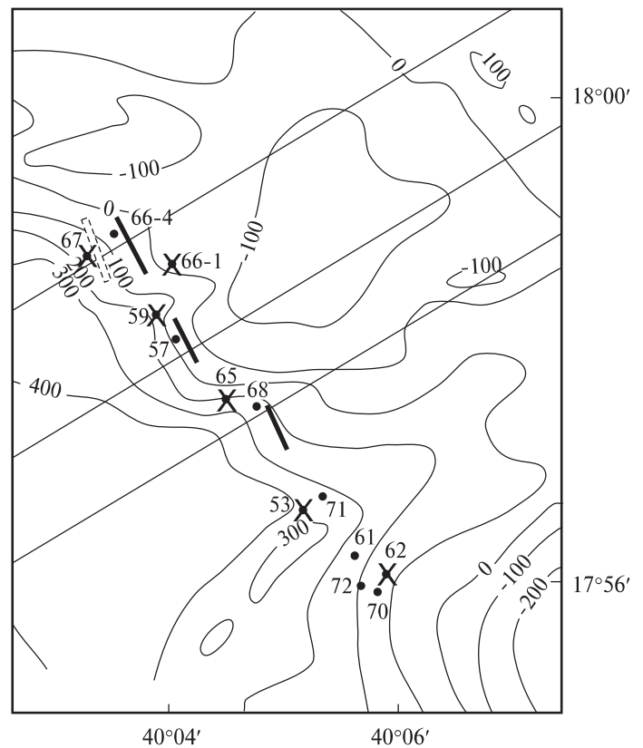
Рис. 3. Карта аномального магнитного поля. Нанесены линии изодинам в нТ, отрезки оси рифта и места отбора образцов базальтов
