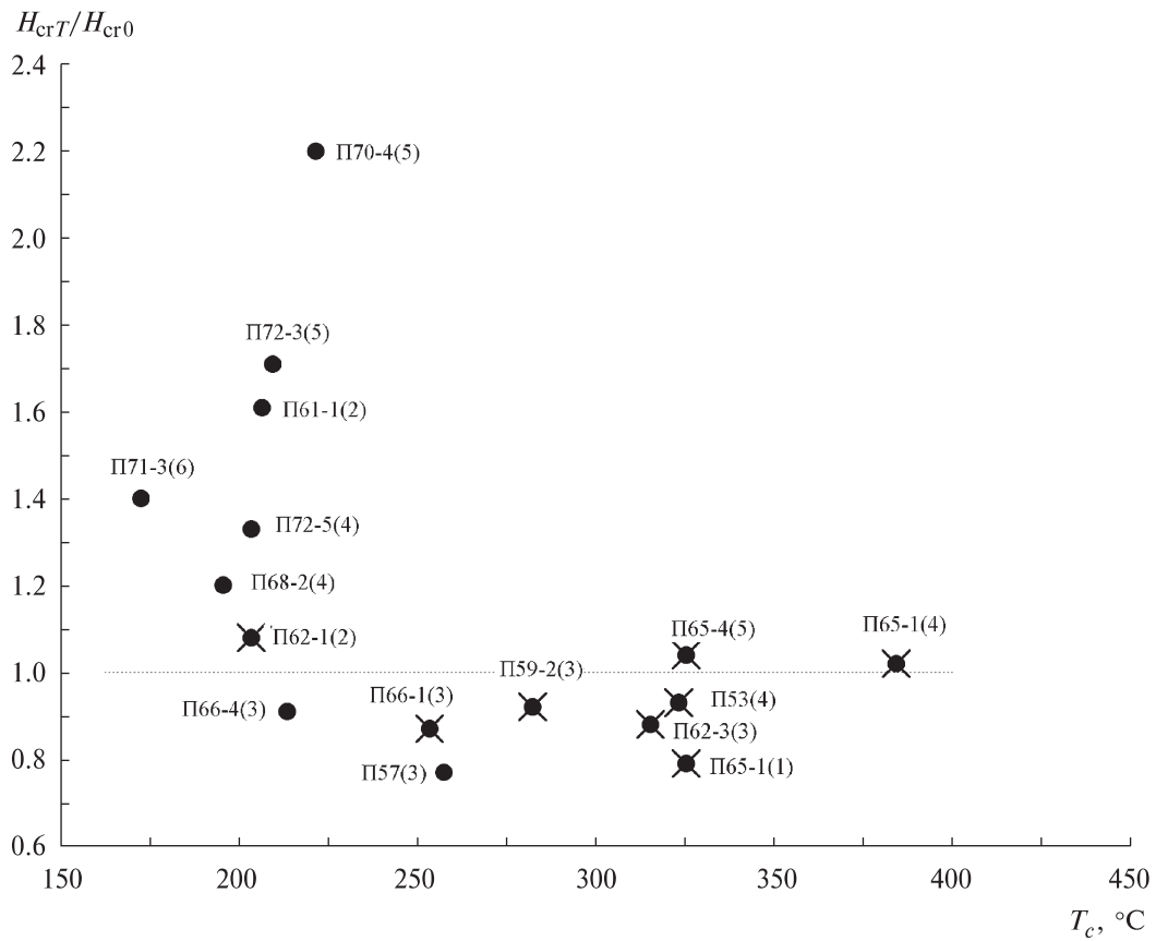
Рис. 5. Изменение остаточно-коэрцитивной силы H_{cr} образцов базальтов с различными температурами Кюри T_c после их нагрева до T = 600^\circ\text{C}
