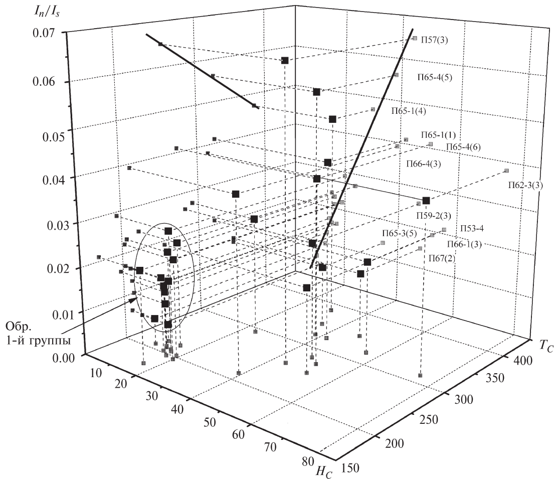
Рис. 4. Нормированная естественная остаточная намагниченность I_n/I_s образцов, имеющих различные величины коэрцитивных сил H_c и температур Кюри T_c
