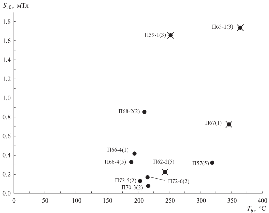
Рис. 6. Соотношение между постоянной магнитной вязкости S_{v0} и температурой блокирования T_b
